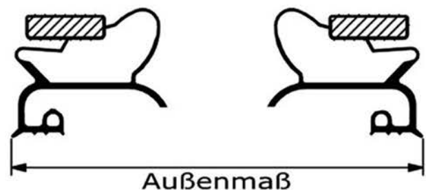
schraubbare Dichtung
