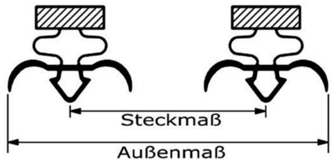
steckbare Dichtung
