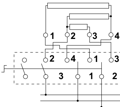
Kochplatte 2x3 Anschlüsse 1x3-poliger Viertaktschalter
