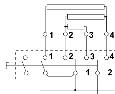
Kochplatte 4 Anschlüsse 2-poliger Siebentaktschalter
