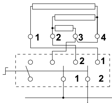
Kochplatte 4 Anschlüsse 2-poliger Fünftaktschalter
