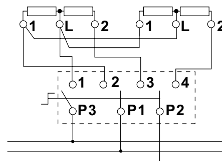
Kochplatte 2x3 Anschlüsse 1x3-poliger Viertaktschalter
