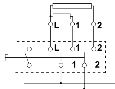
Kochplatte 4 Anschlüsse 2-poliger Fünftaktschalter
