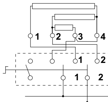
Kochplatte 4 Anschlüsse 2-poliger Viertaktschalter
