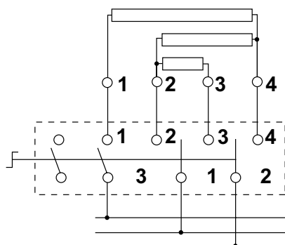
Kochplatte 2x3 Anschlüsse 2x2-poliger Viertaktschalter
