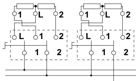
Kochplatte 2x3 Anschlüsse 2x2-poliger Viertaktschalter
